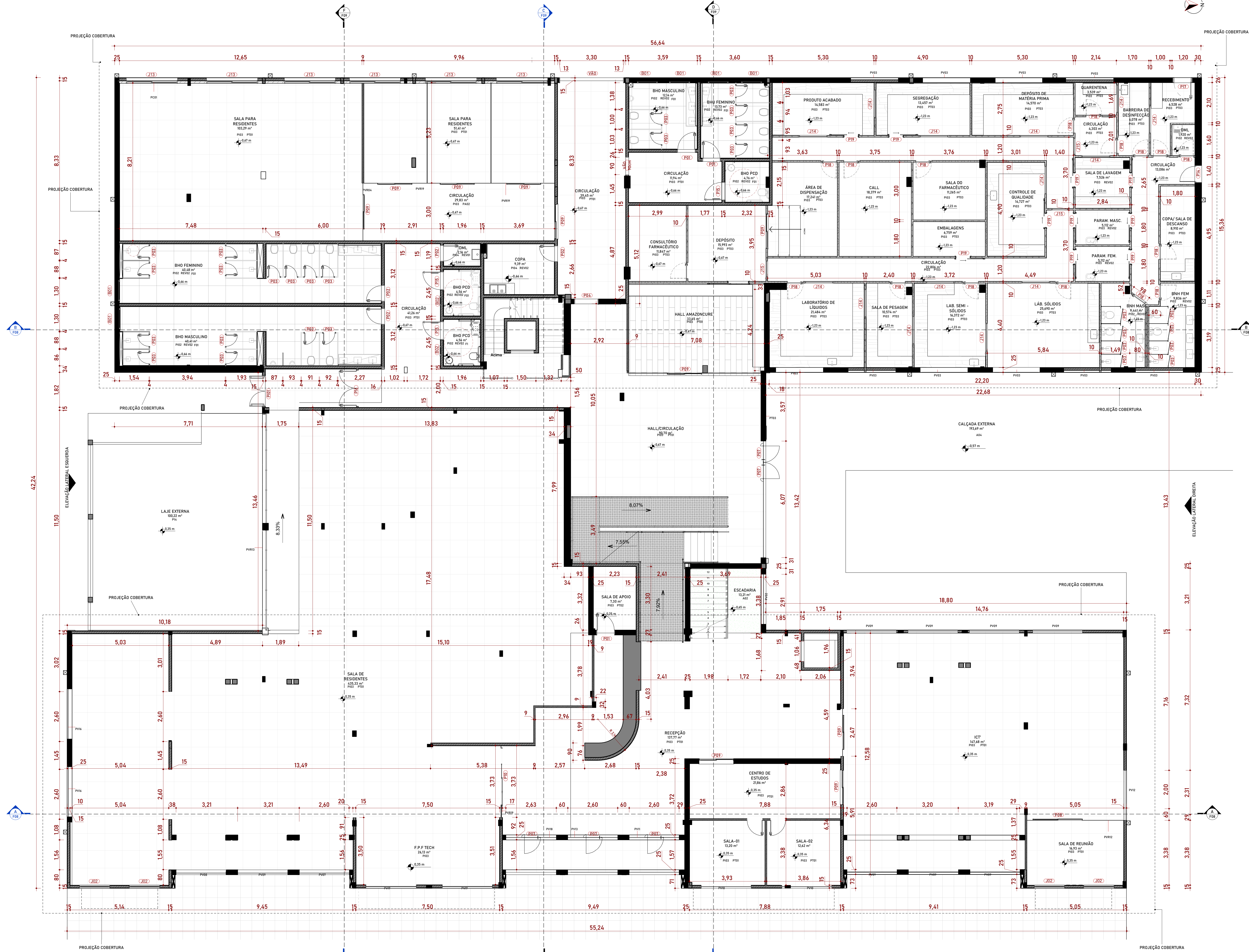
1 PLANTA BAIXA - TÉRREO - BLOCO 01 E 02 1:75
